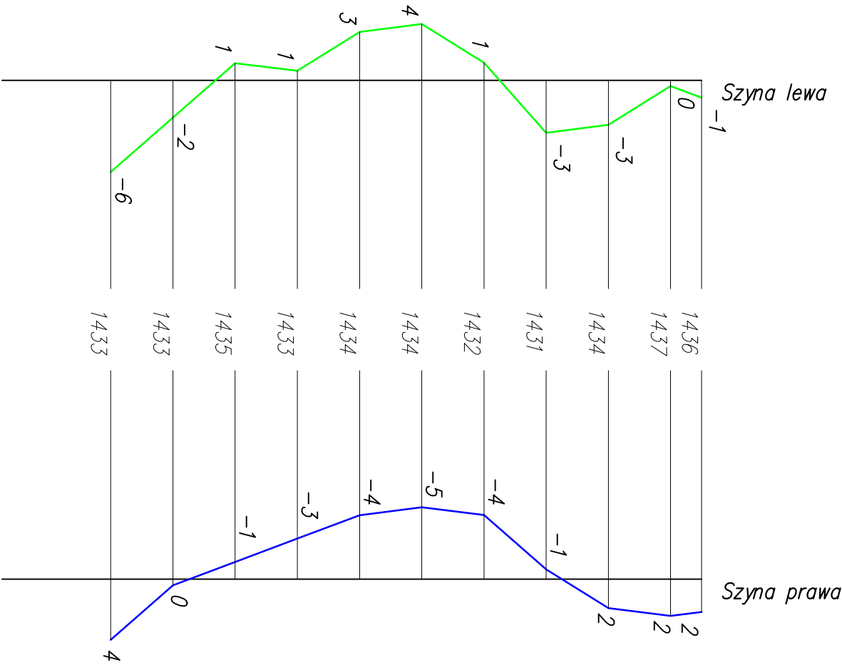
Wykres odkształceń poziomych
